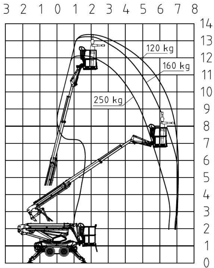
Kuva 4 Ulottumakaavio
