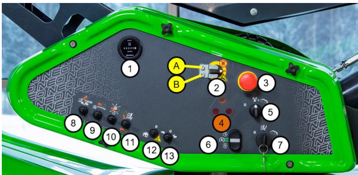
Kuva 8 Alaohjauspaneeli
