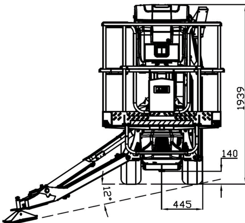
Kuva 3 Päämitat, taka
